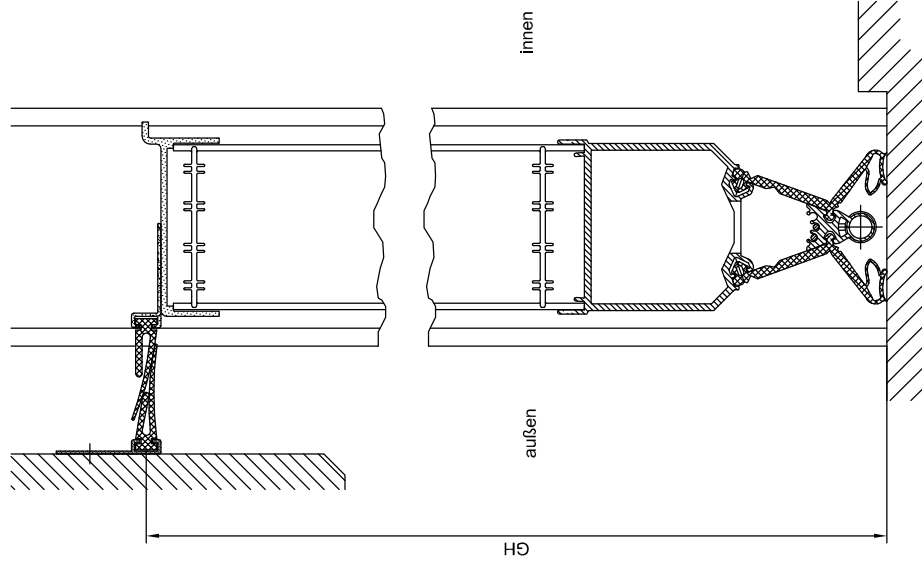
Vertikalschnitt
