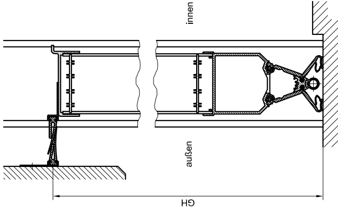
Vertikalschnitt
