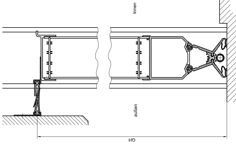
Vertikalschnitt
